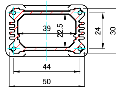
A-A ( 1 : 1.5 )
